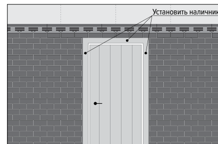
Рис. 7.2. Установка наличников
